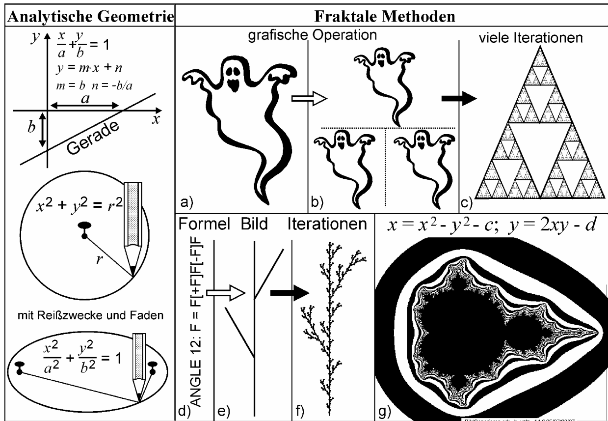
Bild 3. Mittels geometrischer und fraktaler Methoden zum Bild.
