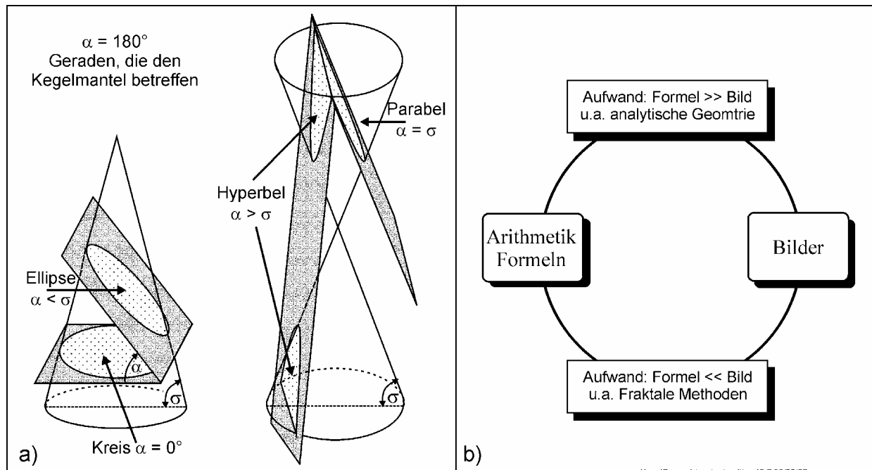
Bild 4a. Bestimmung der Art des Kegelschnitts mit zwei Winkeln \alpha und \sigma sowie b) das Verhältnis von analytischer und fraktaler Geometrie.
